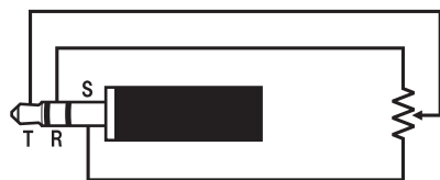
Педаль «экспрессии» типа 2*
